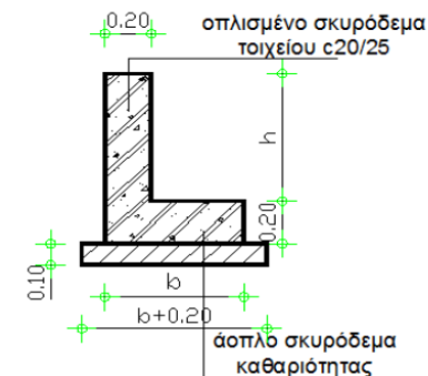
ΕΝΔΕΙΚΤΙΚΗ ΤΟΜΗ ΤΟΙΧΕΙΟΥ ΕΠΙΠΕΔΩΝ
